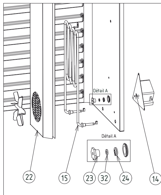
Circuit d'air/ Air circuit
